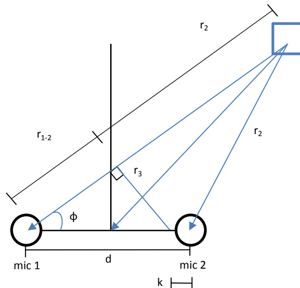
Fig 4.1 Modelo campo cercano del sonido 9
