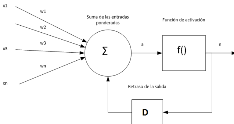
Figura 3.6 Unidad básica de la red neuronal recurrente, neurona feed-back.
