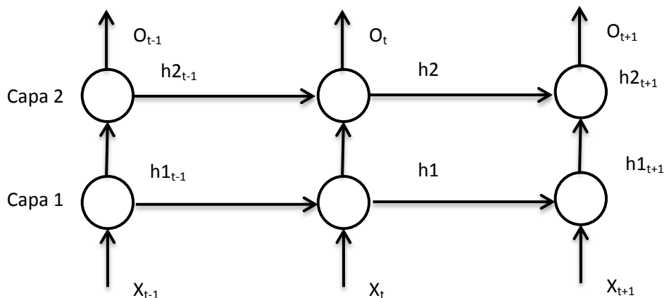
Figura 5.3 Despliegue en el tiempo de la red neuronal recurrente la cual recibe como entrada la STFT de la señal de voz.
