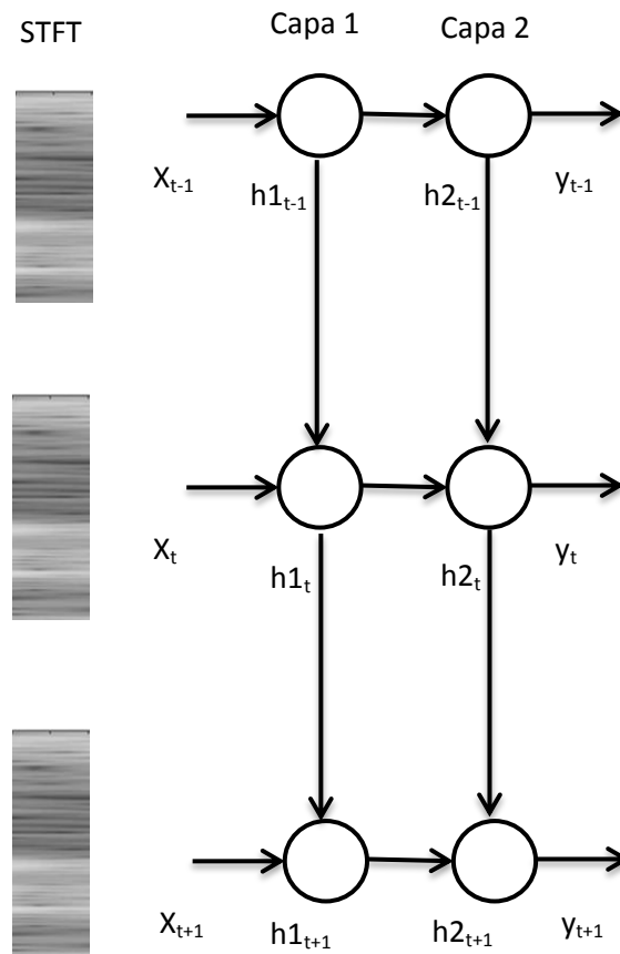
Figura 3.11 Despliegue en el tiempo de la red neuronal recurrente la cual recibe como entrada la STFT de la señal de voz.
