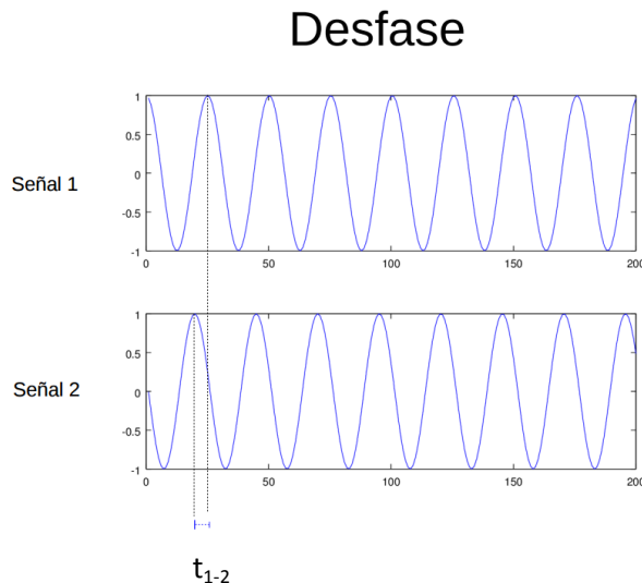
Fig 4.3 Desfase de una misma señal en diferentes sensores 11
