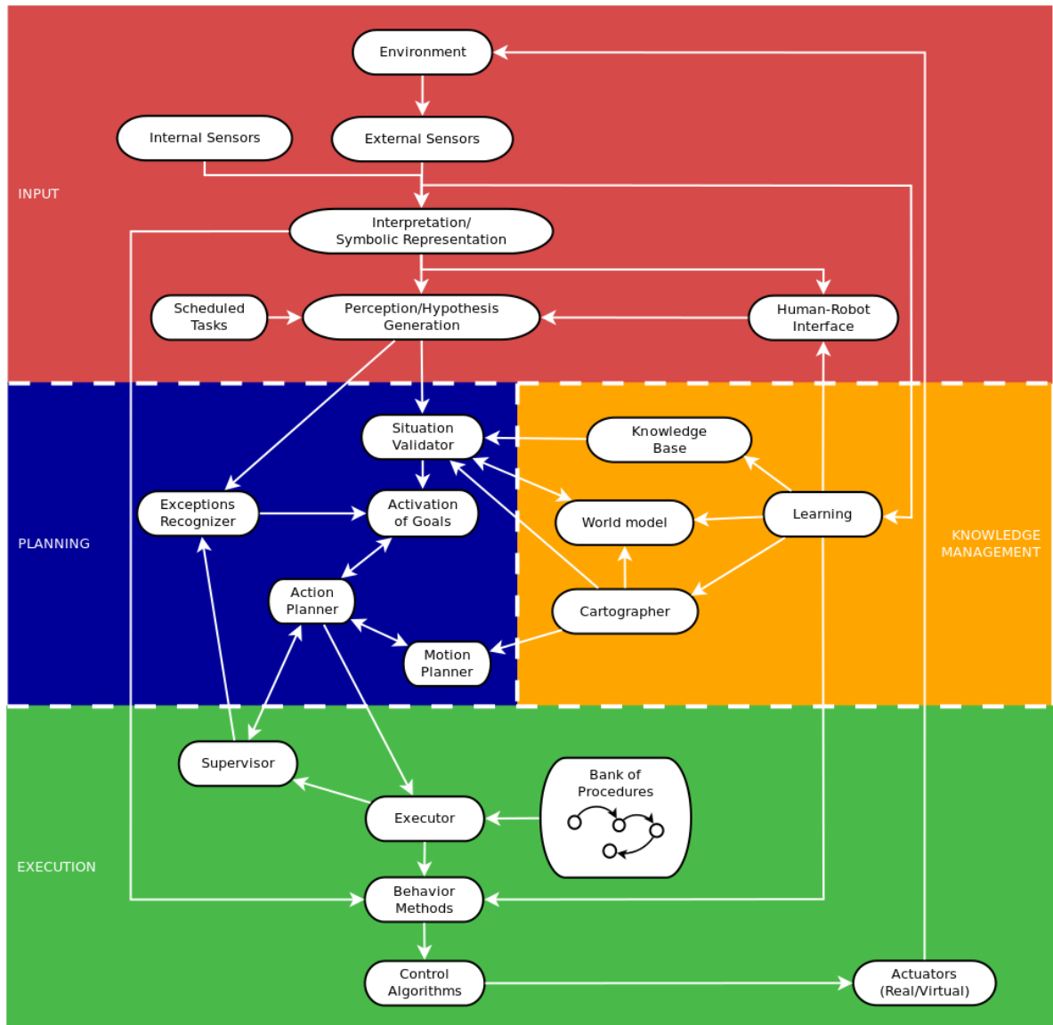
Figura 1.1 Diagrama de los sistemas del Robot Justina (VirBot versión 2016).
