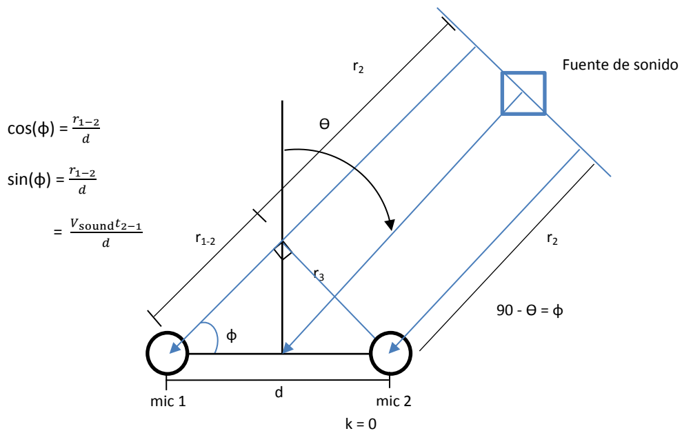
Fig 4.2 Modelo campo cercano del sonido 1
