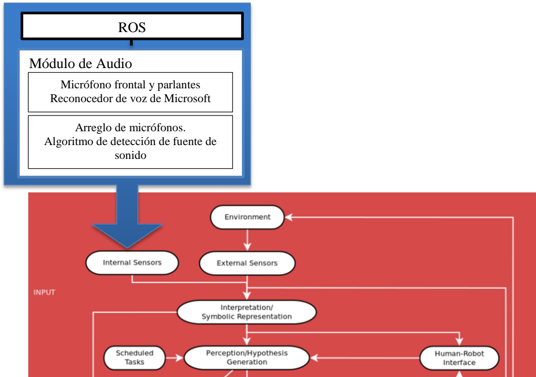
Fig. 5.4 Actualización del robot con el módulo de detección de fuente de sonido (sistema actualmente en 2017).
