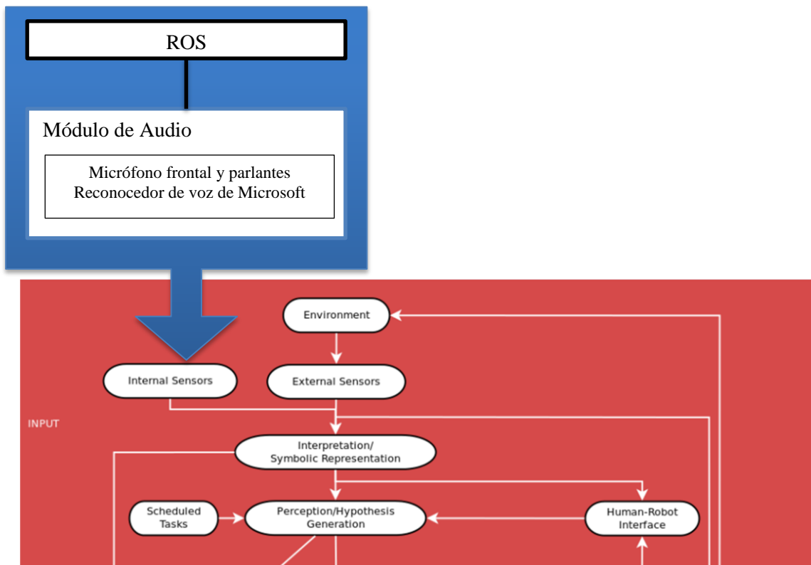
Figura 1.2 Diagrama de los sistemas de entrada del Robot Justina, se muestra parte de los sensores de entrada actuales (VirBot versión 2016).
