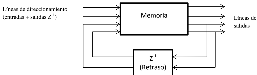
Figura 3.12 Direccionamiento de memoria usando entradas al sistema y parte de las salidas del estado presente
