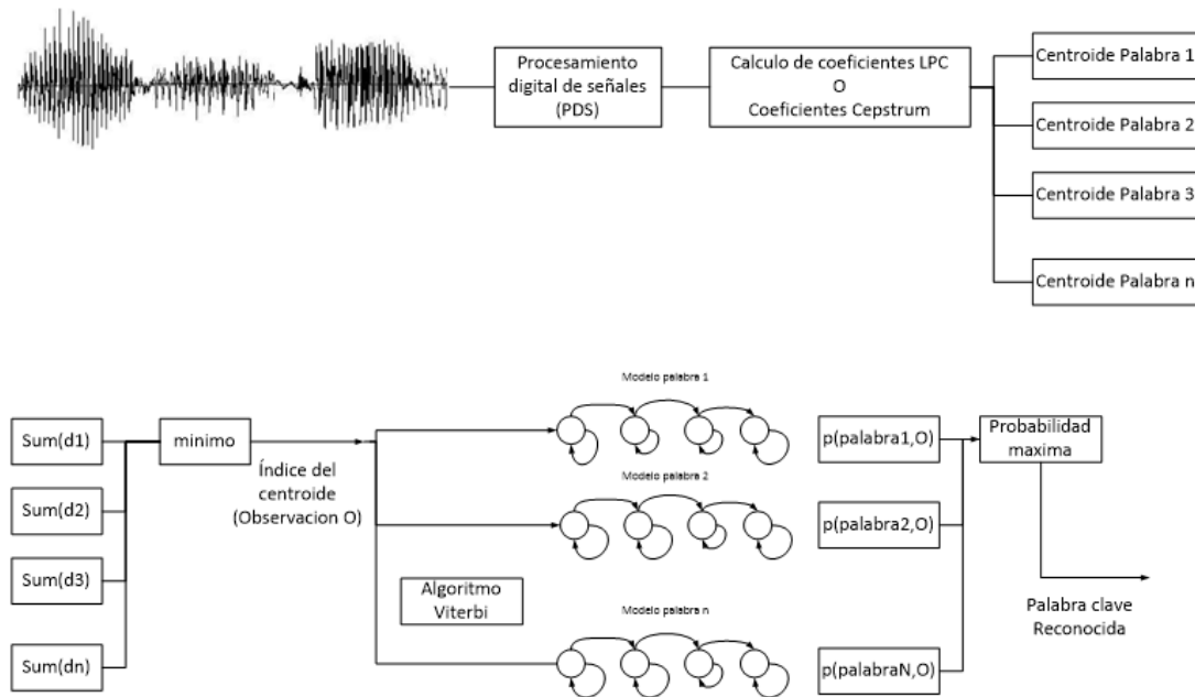
Figura 2.5 Sistema convencional de reconocimiento de palabras claves en una trama de voz, de izquierda a derecha el flujo es el mismo al de la figura 2.2 con la adición de HMM para determinar la palabra clave.
