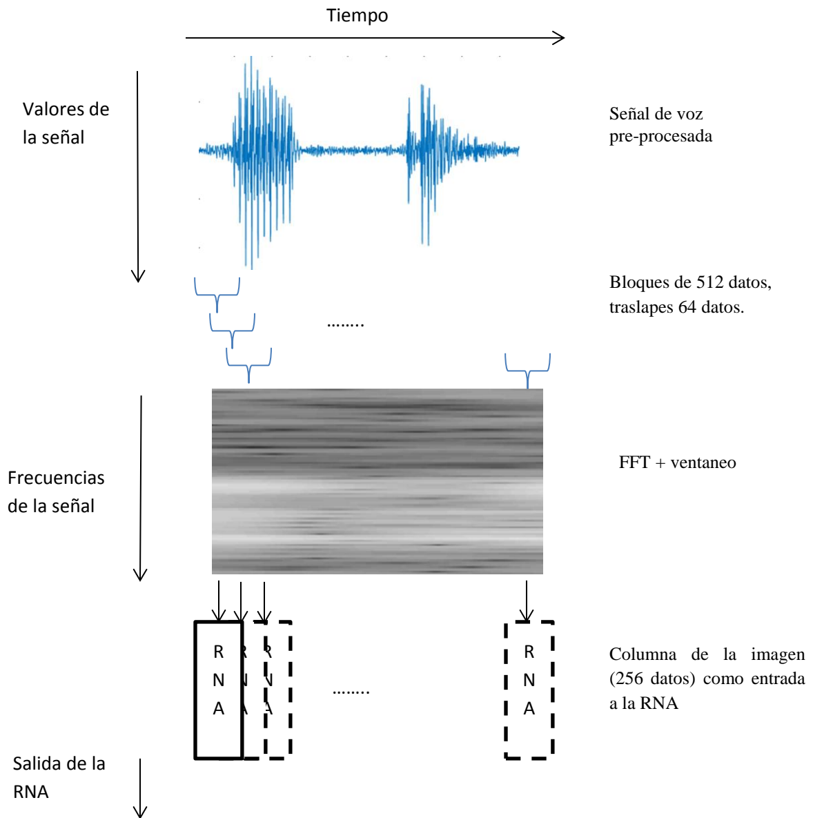
Figura 3.10 Metodología para alimentar la señal de voz a la red neuronal
