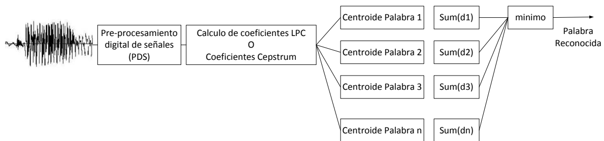
Figura 2.3 Sistema de reconocimiento de palabras aisladas, digitalización de la señal, procesamiento y acondicionamiento de la misma, etapa de codificación y descripción, distancias con centroides de patrones en previo entrenamiento y finalmente selección de la palabra.
