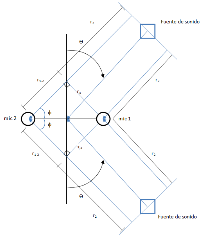
Fig 4.6 Posibles soluciones para un arreglo lineal
