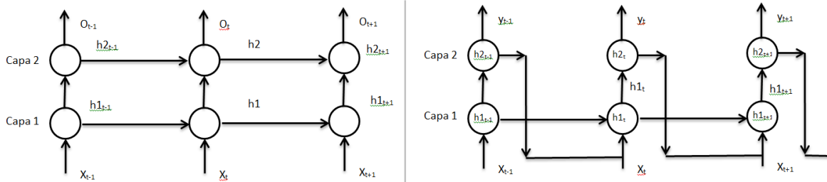
Fig 5.1 Arquitectura de las redes recurrentes utilizadas, a la izquierda el modelo convencional de redes recurrentes (A y B) y a la derecha la propuesta de red basada en máquina de estados (C).
