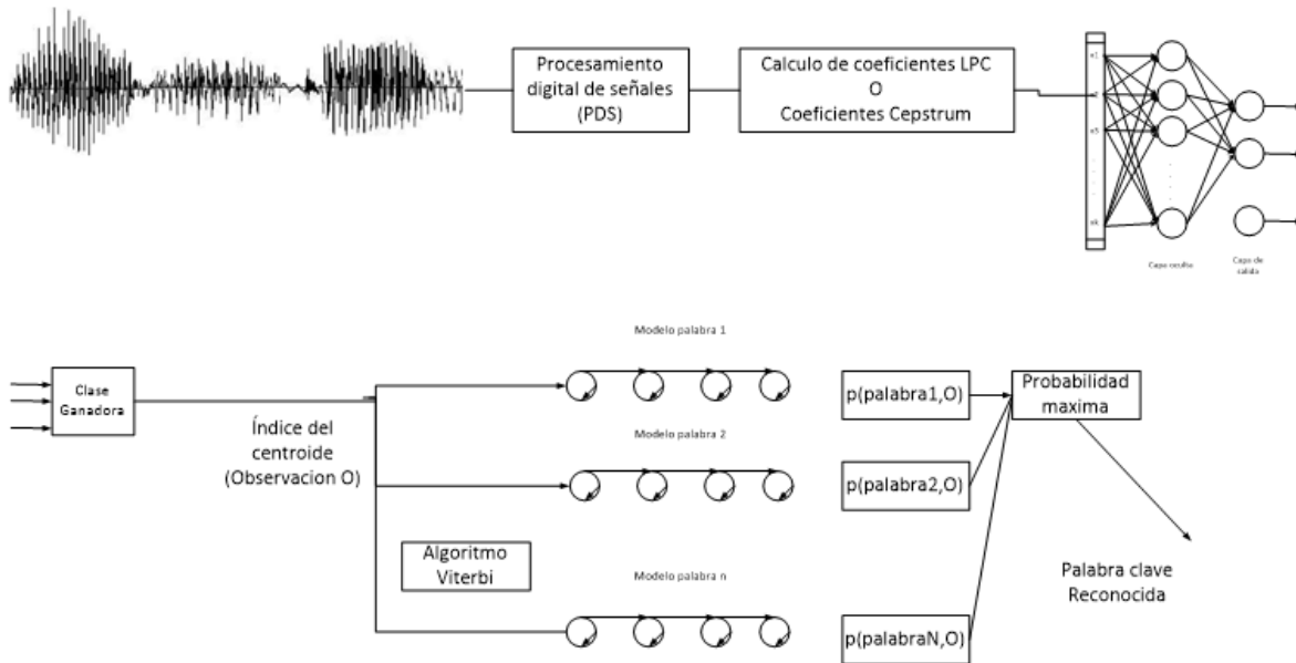
Figura 2.6 Sistema de reconocimiento de palabras clave en una trama de voz utilizando un clasificador por redes neuronales multicapa de los descriptores LPC o Cepstral y a la salida de la red neuronal se selecciona la clase ganadora al cual pertenece el fonema o silaba siendo la observación para HMM.
