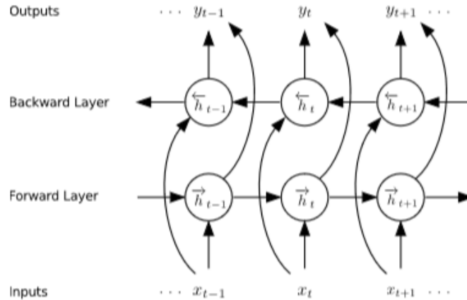
Figura 3.4 Arquitectura BRNN 5
