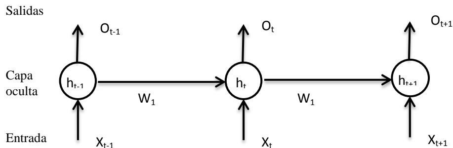
Figura 3.3 Arquitectura FRNN
