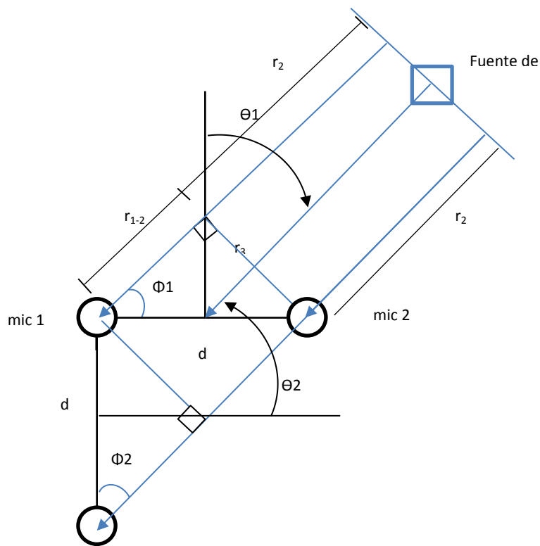
Fig 4.7 Arreglo de micrófonos propuesto.
